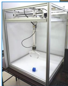
4軸クレーン装置
